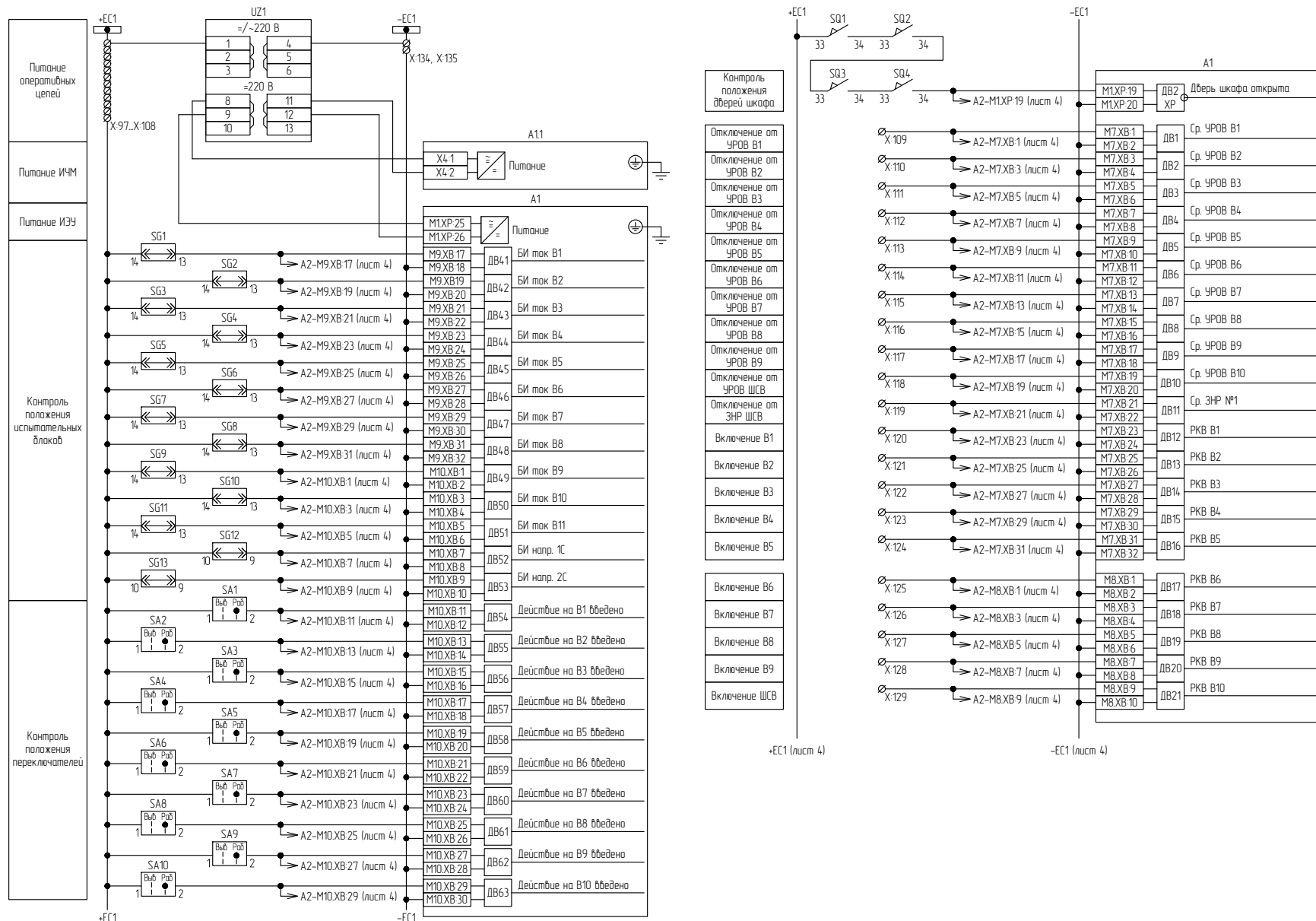
Цени оперативного тока
